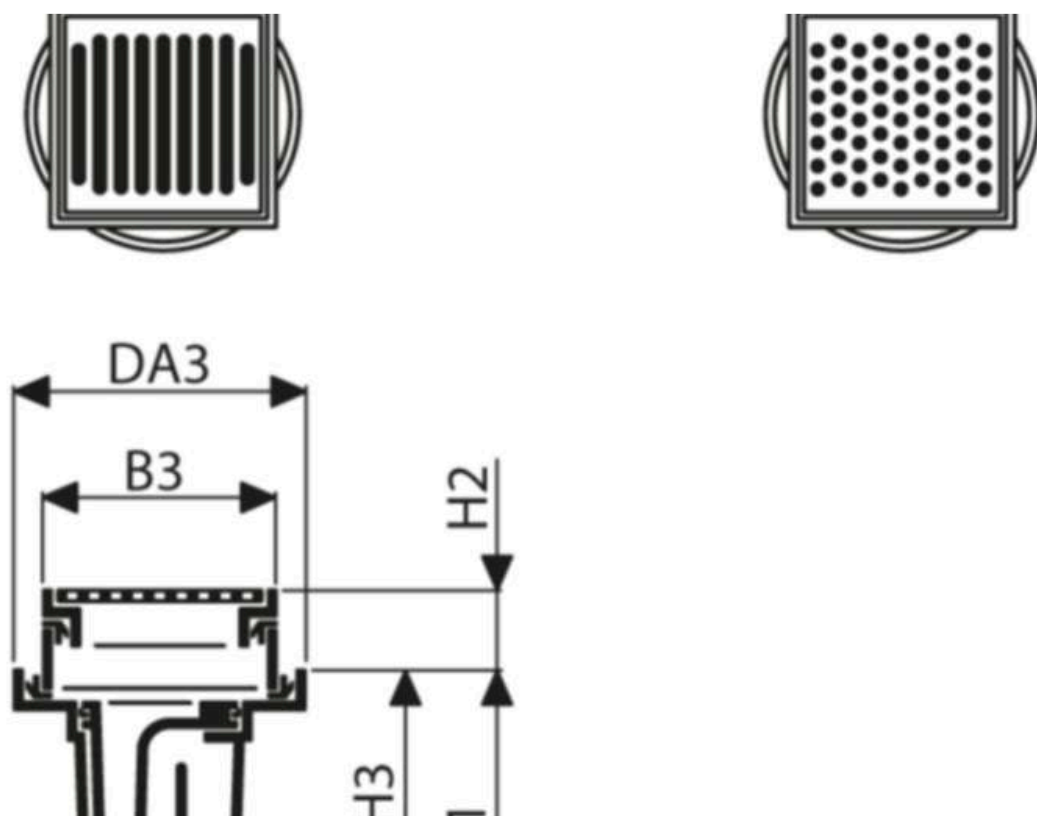
Siphon de sol - Figure 1660-106-20 avec grille INOX
