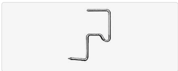
Crampon tempête no 1 Ø3,5 mm cuivre NEO 5051.100 pour tuile plate ref. 186 0.20 CHF HT la pièce au lieu de 0.71 stock 500 pièces
