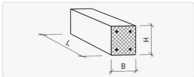
Linteau béton épaisseur 20 cm 155x20x14
