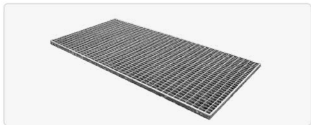
Grille-caillebotis pour saut-de-loup, praticable, CREA, 210 X 81
