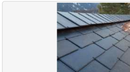
Ardoise fibro-ciment Alpina 60/40 cm ép.4mm noir-bleuté (10.4 pces/m2)
