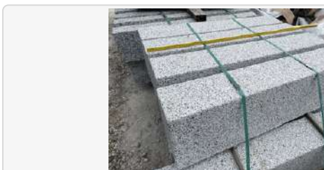
Bordure, granit blanc UE franchissable, faces vues grenillées
