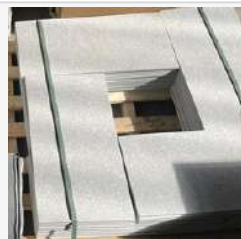
S-302 Dalle, quartzite blanche, surface flammée et brossée, dim. 30x60cm.
