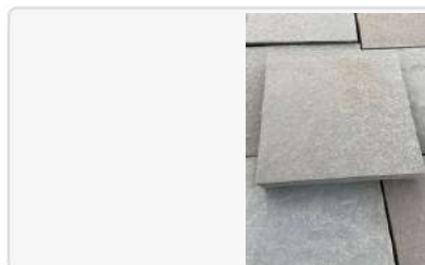
Dalle, grès Dinara, surface flammée et brossée, dim. 20x20cm, épaisseur 3cm
