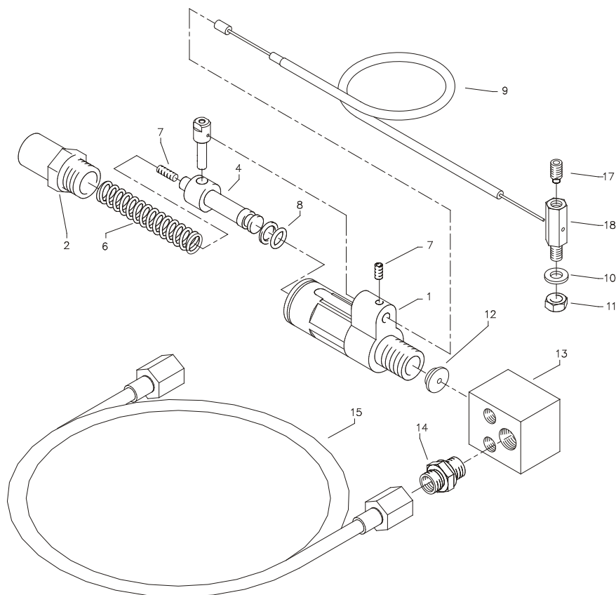
Liste des pièces de rechange Kränzle B230 T / B240 T / B270 T Régulateur de vitesse
