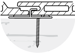
FIXATION PAR CLIP
