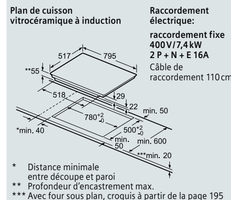
EH845BFB1E Dimensions en mm
