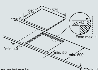
Plan de cuisson vitrocéramique à induction
