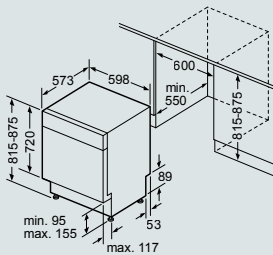
SE43HS36TE Dimensions en mm
