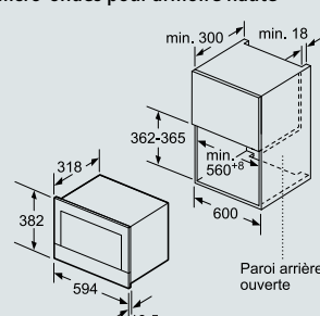
Micro-ondes pour armoire haute
