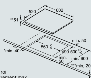
Plan de cuisson vitrocéramique à induction
