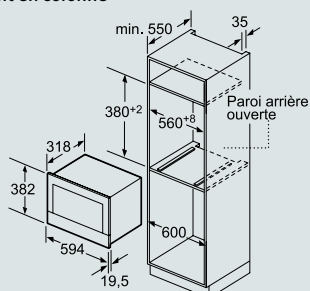
Micro-ondes pour encastrement en colonne
