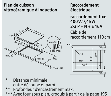
EH801FVB1E Dimensions en mm
