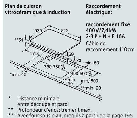
EH875FVB1E Dimensions en mm
