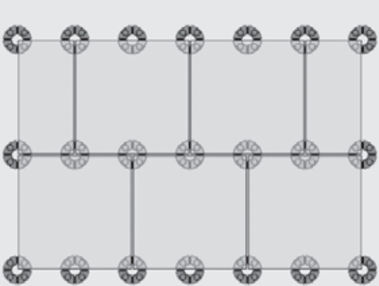
60x60 POSE DÉCALÉE 60x60 STAGGERED INSTALLATION 60x60 VERSETZTE VERLEGUNG
