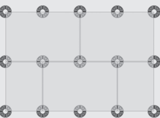
60x90 cm POSE DÉCALÉE 60x90 cm STAGGERED INSTALLATION 60x90 cm VERSETZTE VERLEGUNG
