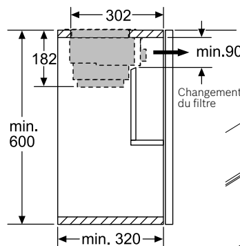
installation dans un meuble haut
