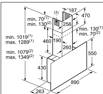
(1) Évacuation d'air (2) Circulation d'air (3) Sortie de l'air - remettre les fentes vers le bas lors de l'évacuation d'air
