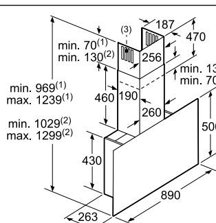
(1) Évacuation d'air (2) Circulation d'air (3) Sortie de l'air - remettre les fentes vers le bas lors de l'évacuation d'air
