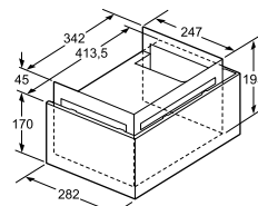
Monté à l'intérieur du canal
